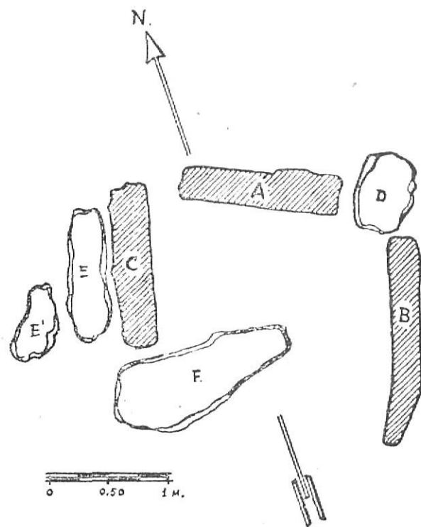
Fig. 3. — Planta del dolmen de La Castellana según F. Riu. Las piedras A, B y C son las que quedan in situ.
