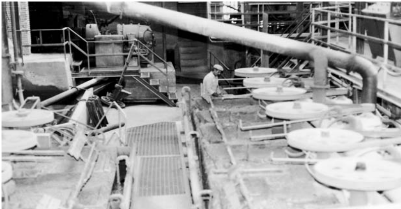
Cel·les de flotació d'espat fluor de la planta de concentració de mineral de les Mines d'Osor. Fotografia feta durant el mes d'agost de l'any 1979.
