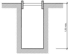
Rasa sense apuntalament
