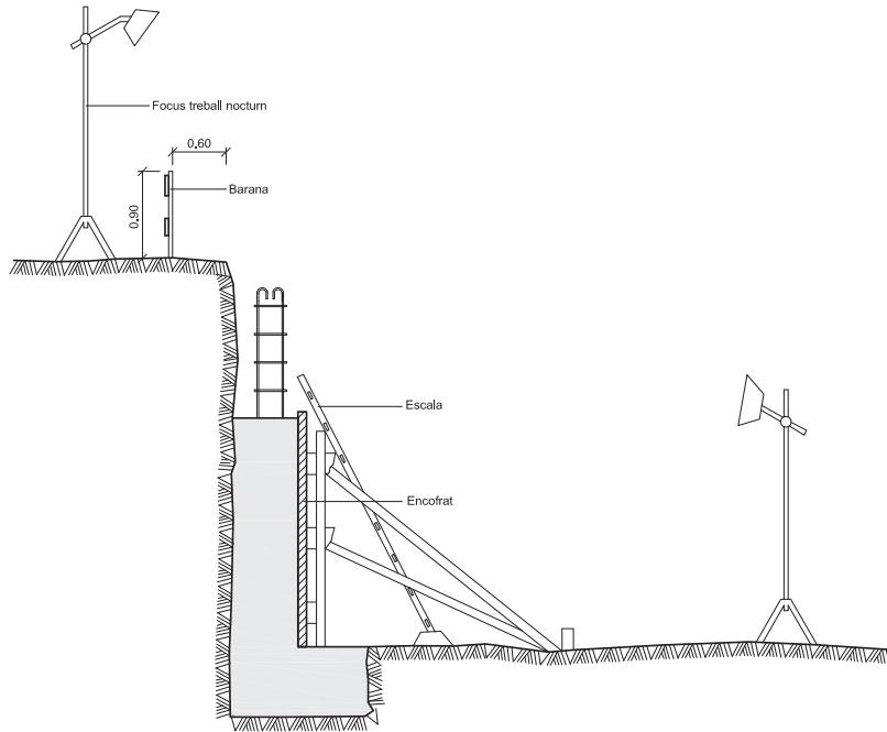
DETALL 010203 Protecció per a murs de contenció
