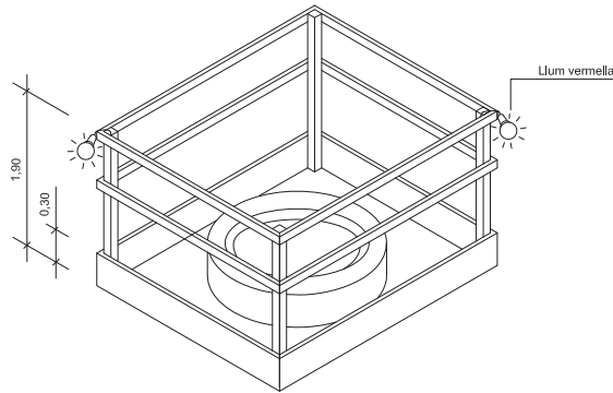
DETALL 010207 Proteccions en forats i obertures Isomètrica
