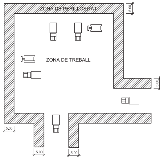
DETALL 020100 Delimitació zones de treball ESCALA S/E
