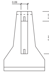
ALÇAT TRANSVERSAL
