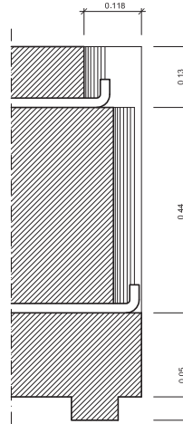
SECCIÓ B-B' ESCALA 1:5
