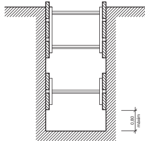
Rases amb apuntalament sense sobrecàrrega
