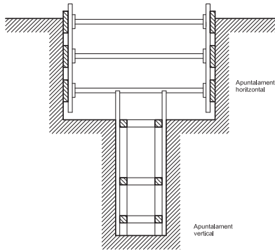
Rasa profunditat amb sobrecàrrega
