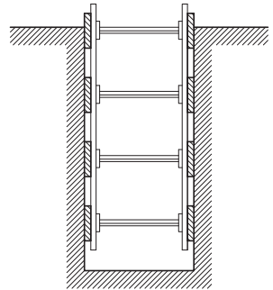
Rases amb apuntalament per sobrecàrrega
