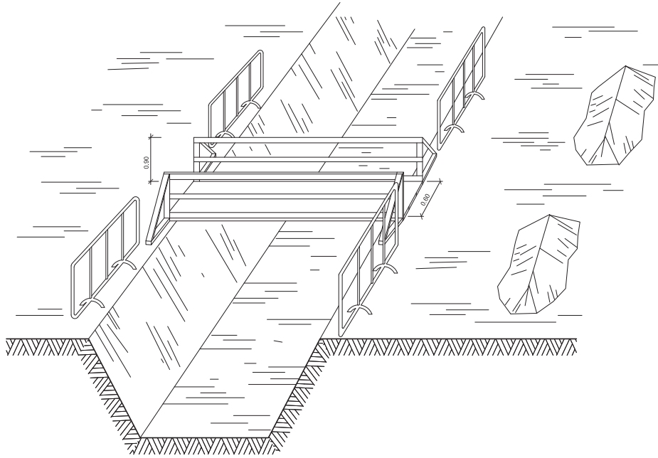
DETALL 010200 Esquema de protecció de rases
