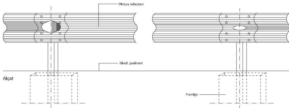
DETALL 010102 Tanca doble ona, tancament d'obra ESCALA 1:5
