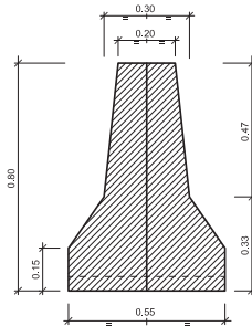
SECCIÓ A-A'
