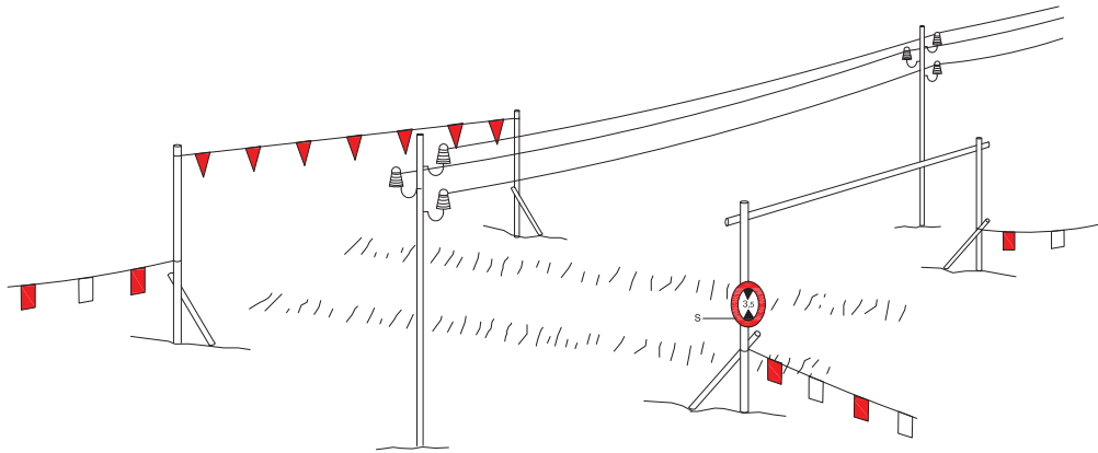
DETALL 010204 Pòrtic de balisament protecció de línies elèctriques aèries
