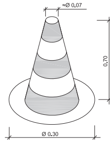
Con de balisament
