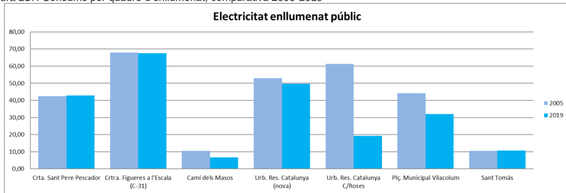
Figura 217. Consums per quadre d'enllumenat, comparativa 2005-2019
