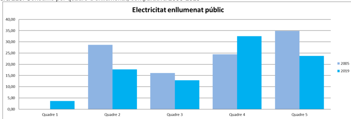
Figura 219. Consums per quadre d'enllumenat, comparativa 2005-2019
