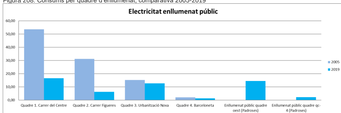
Figura 208. Consums per quadre d'enllumenat, comparativa 2005-2019
