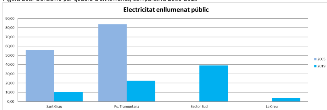
Figura 203. Consums per quadre d'enllumenat, comparativa 2005-2019
