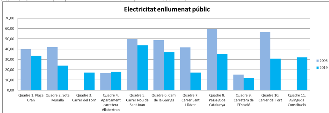
Figura 213. Consums per quadre d'enllumenat, comparativa 2005-2019
