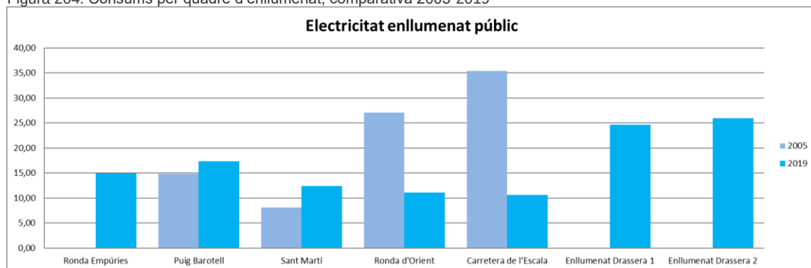
Figura 204. Consums per quadre d'enllumenat, comparativa 2005-2019
