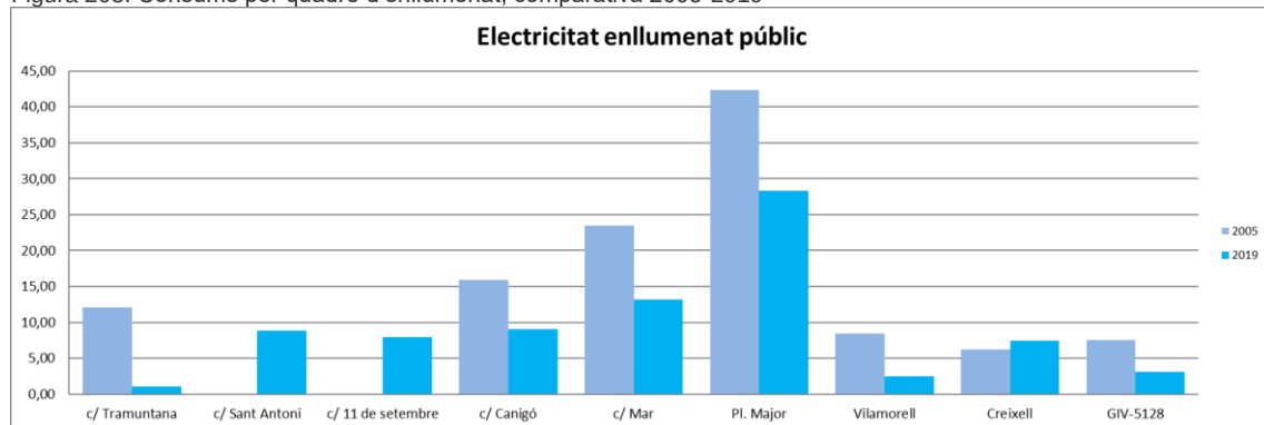
Figura 205. Consums per quadre d'enllumenat, comparativa 2005-2019
