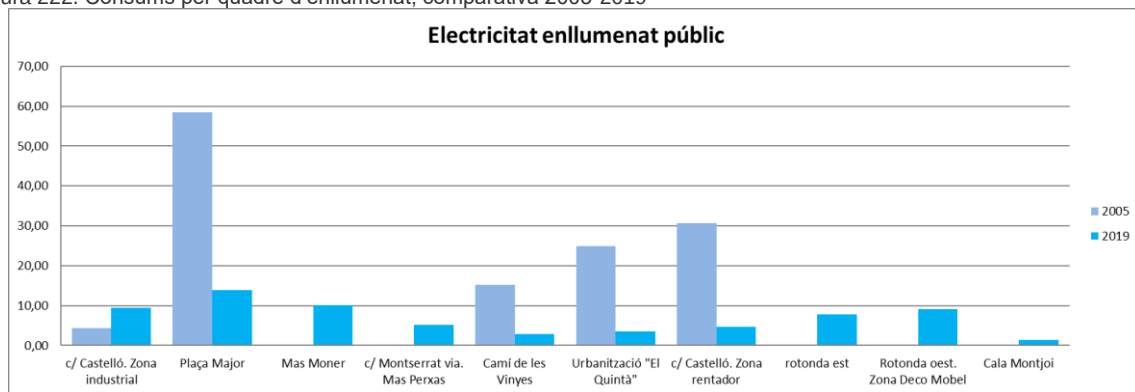
Figura 222. Consums per quadre d'enllumenat, comparativa 2005-2019
