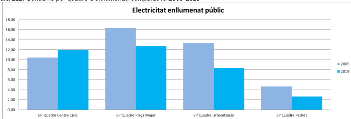
Figura 212. Consums per quadre d'enllumenat, comparativa 2005-2019
