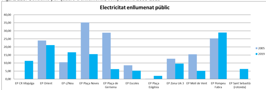
Figura 210. Consums per quadre d'enllumenat, comparativa 2005-2019
