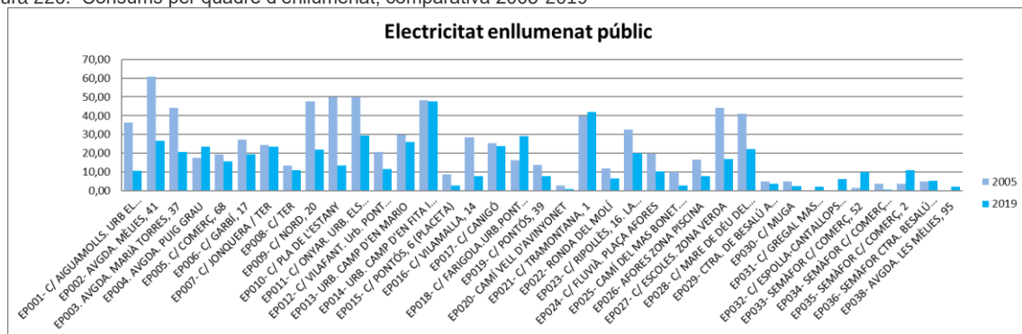
Figura 220. Consums per quadre d'enllumenat, comparativa 2005-2019
