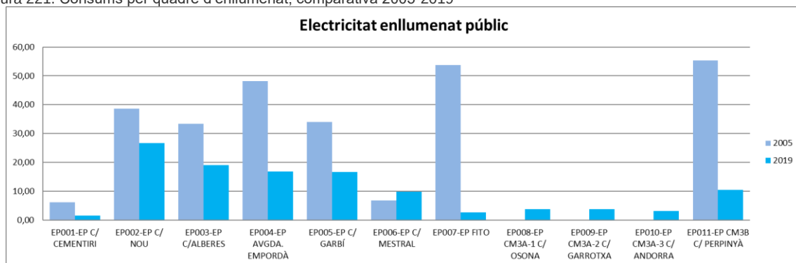
Figura 221. Consums per quadre d'enllumenat, comparativa 2005-2019
