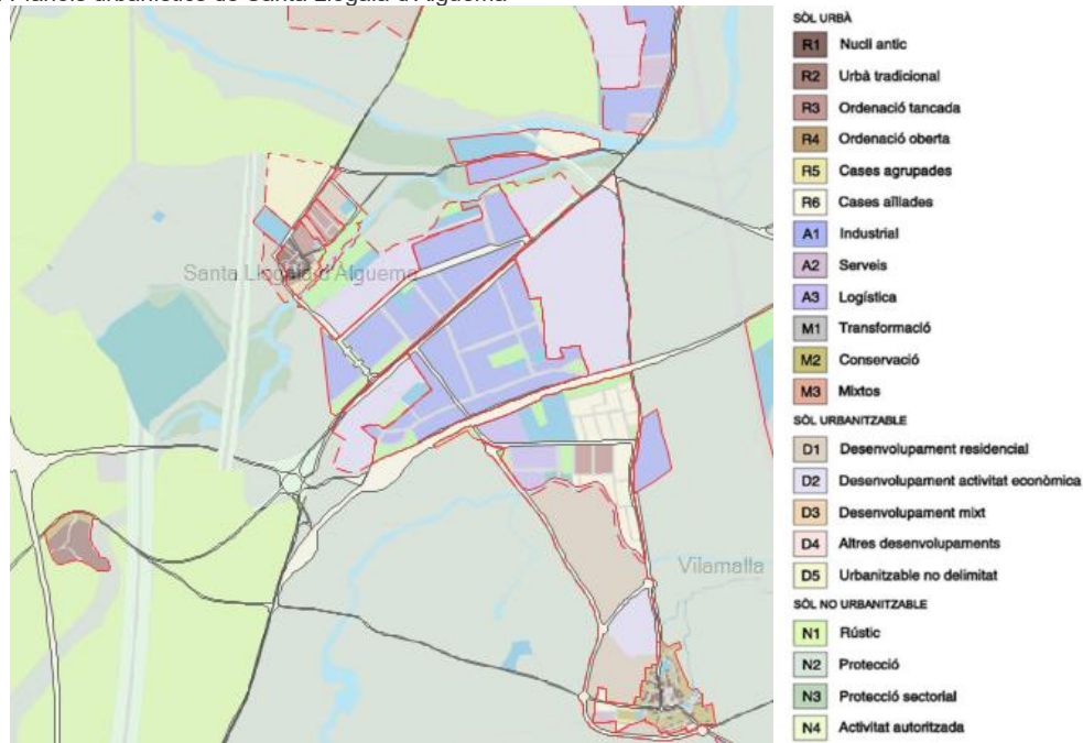
Figura 146. Plànols urbanístics de Santa Llogaia d'Àlguema
