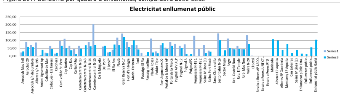
Figura 207. Consums per quadre d'enllumenat, comparativa 2005-2019
