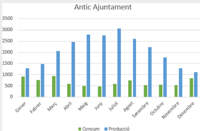
Figura 8. Representació gràfica consum vs. producció Antic Ajuntament Font: Elaboració pròpia
