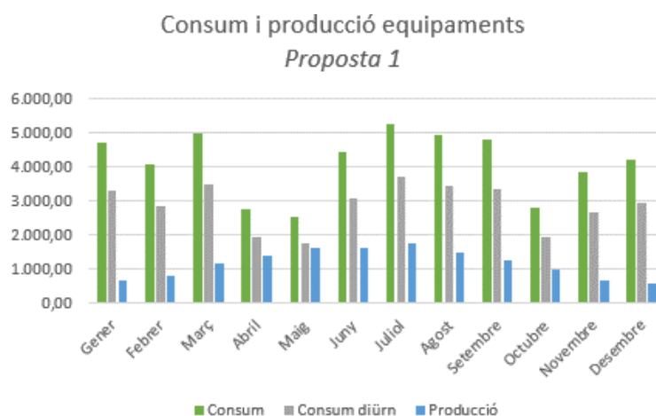
Figura 23. Gràfic consum i producció equipaments municipals Proposta 1
