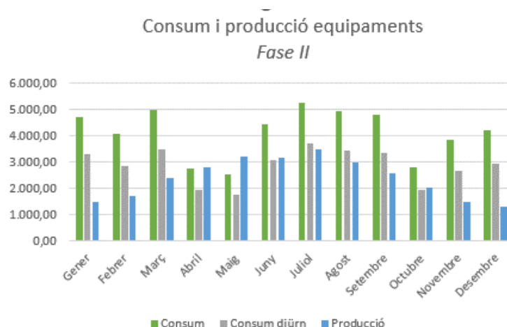
Figura 28. Gràfic consum i producció equipaments municipals Fase II Font: Elaboració pròpia
