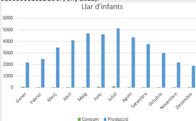
Figura 11. Representació gràfica consum vs. producció Llar d'Infants Font: Elaboració pròpia
