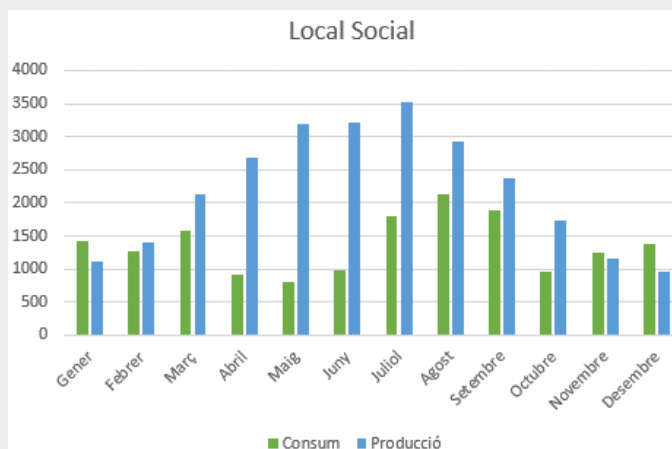
Figura 14. Representació gràfica consum vs. producció Local Social Font: Elaboració pròpia
