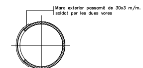
DETALL MARC DE REFORÇ EXTERIOR
