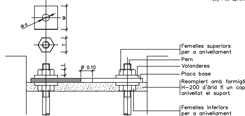
Detall ancoratges de les columnes i bàculs
