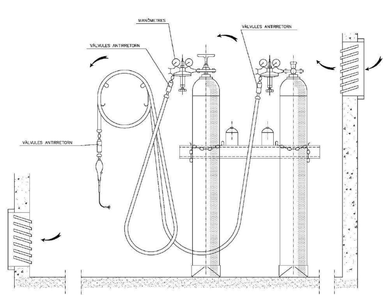
INSTAL·LACIÓ DE BOMBONES D'OXIGEN I ACETILÈ
