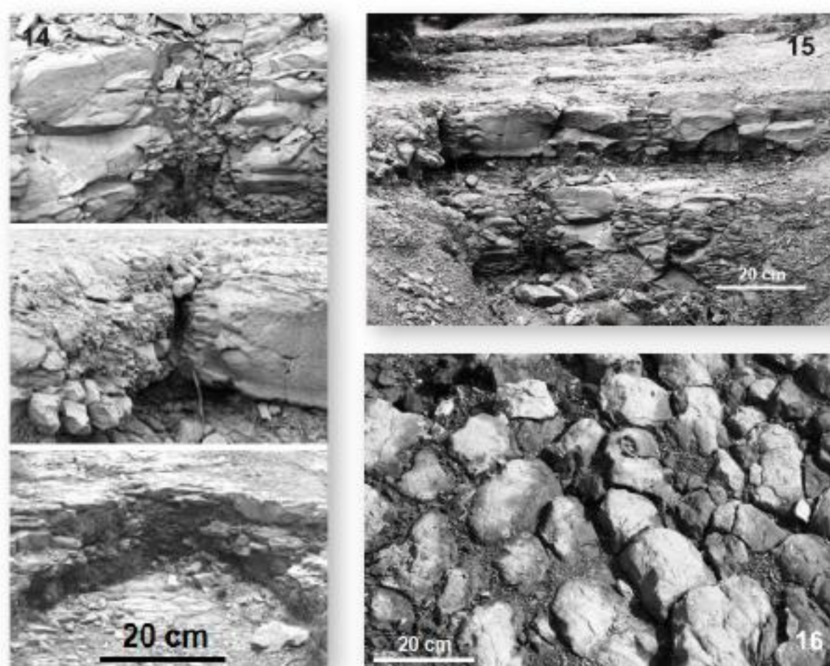
(Fig.14 Formació d'un regueró en el xaragall (secció) (Fig.15 Formes esglaonades) (Fig.16 Disjunció bolar)
