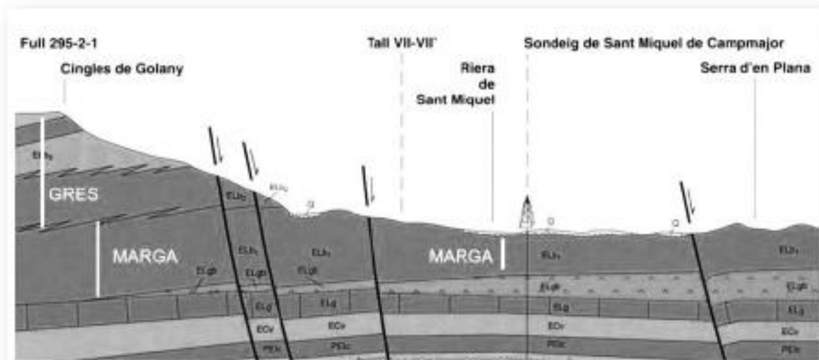
(Fig.6 Tall geològic. Serra de la Cadamont 1:25000 ICGC)
