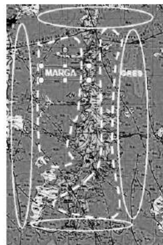
(Fig.5 Mapa geològic 1:25000 ICGC)
