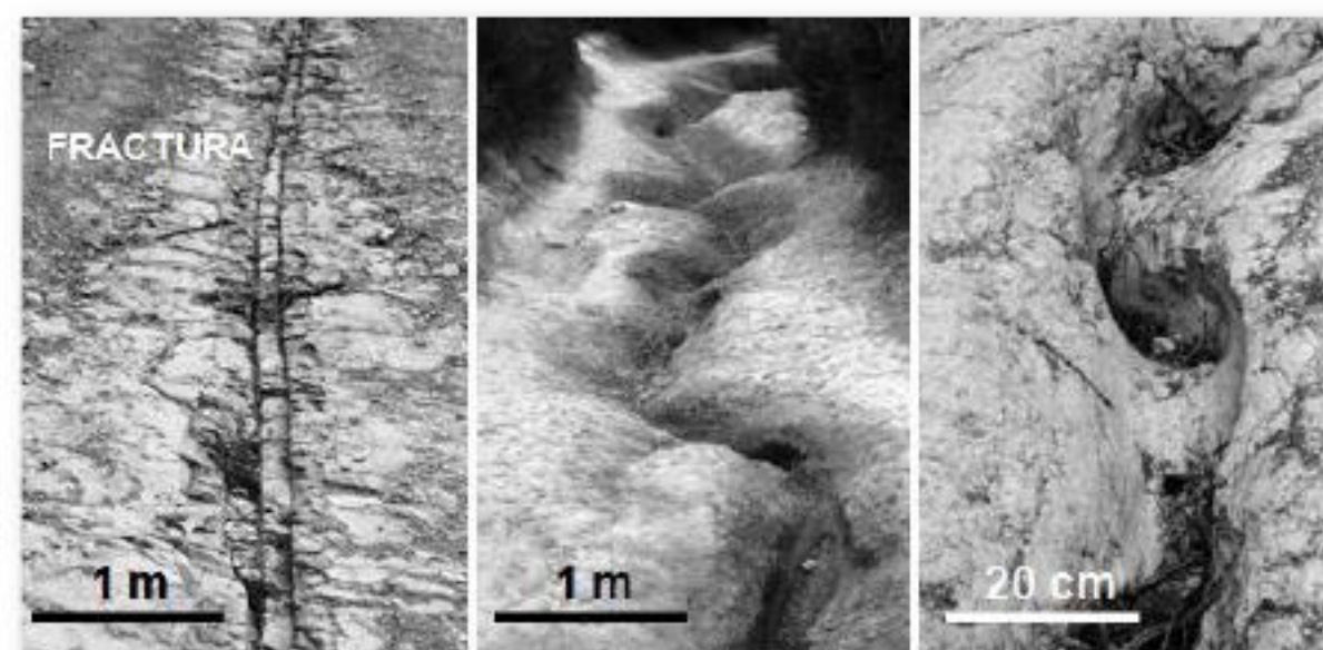
(Fig.13 Formació d'un regueró en el xaragall (planta)
