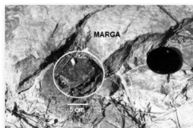
(Fig.9 Nòdul de pirita in situ)
