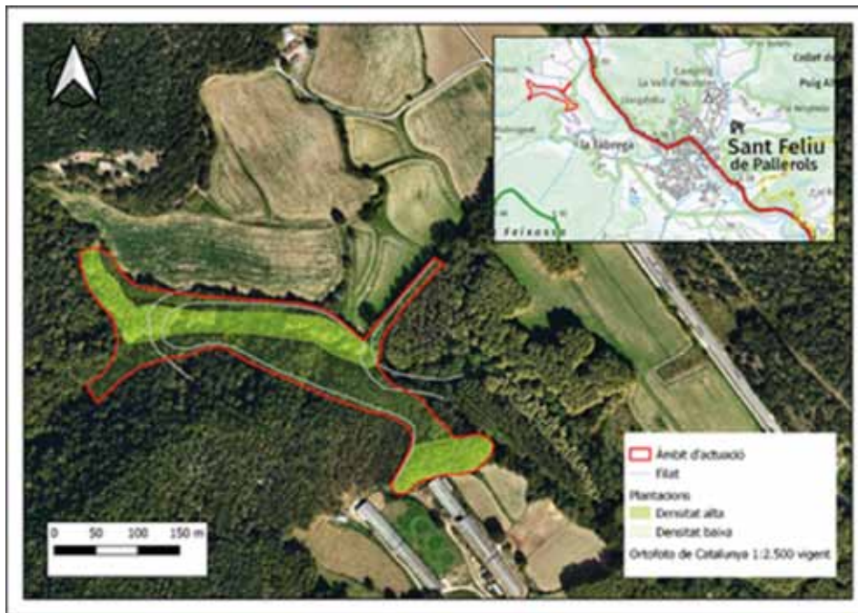
Figura 2. Plànol del projecte de recuperació del bosc de ribera al torrent del Mosquer
