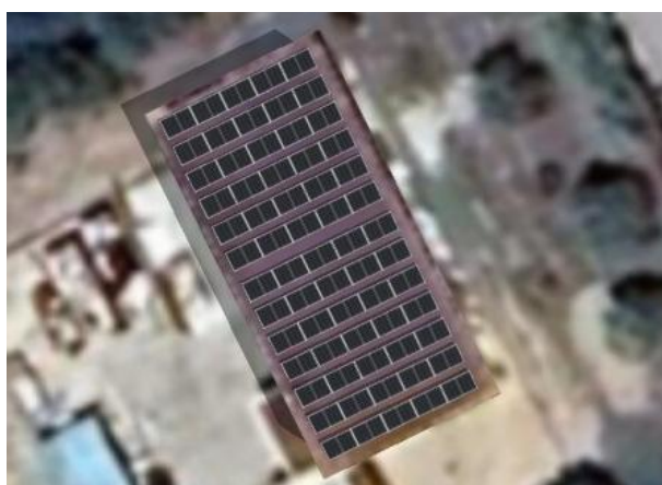
Figura 9. Imatge en 3D de la instal·lació FV 2 plantejada. Font: PVSOL.
