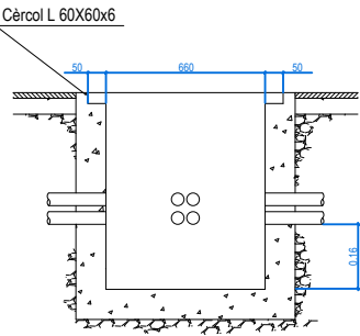
SECCIÓ B-B'
