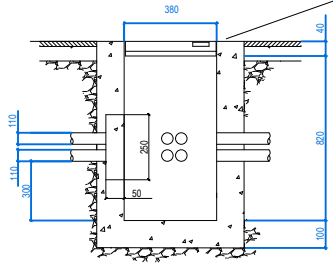
SECCIÓ A-A'
