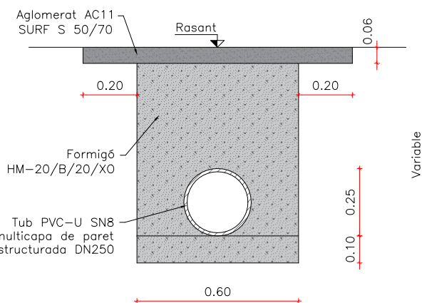
DETALL RASA CLAVEGUERAM TIPUS 2 Esc 1/20
