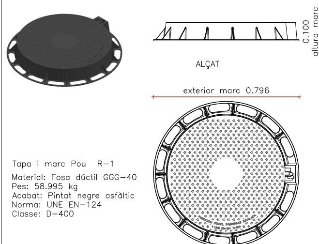
DETALL TAPA I MARC AMB TANCA DE BLOQUEIG I JUNTA D'INSONORITZACIÓ Esc 1/20
