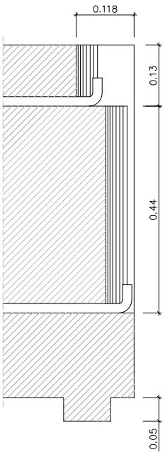
SECCIÓ B-B'
