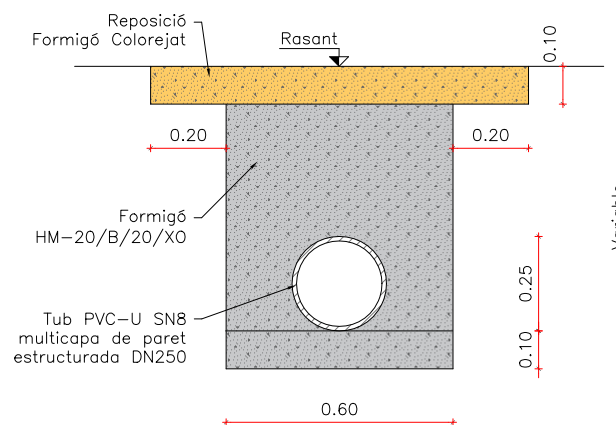
DETALL RASA CLAVEGUERAM TIPUS 3 Esc 1/20
