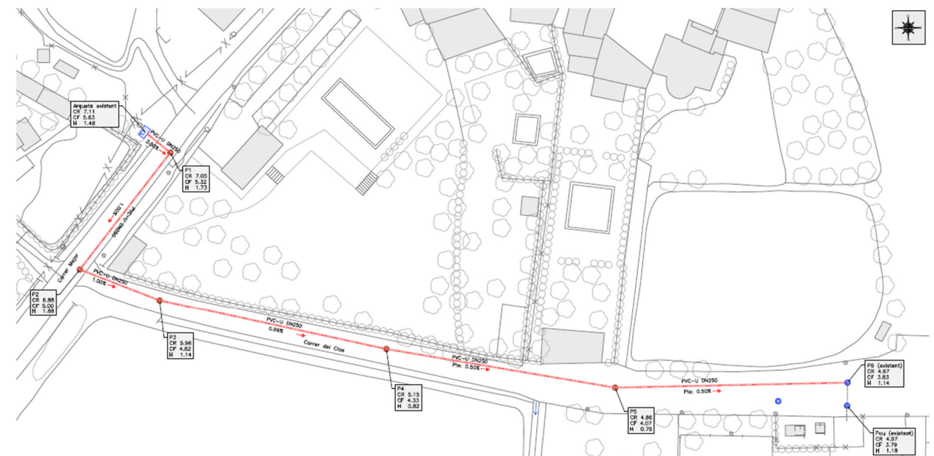
Figura 4. Planta proposada
