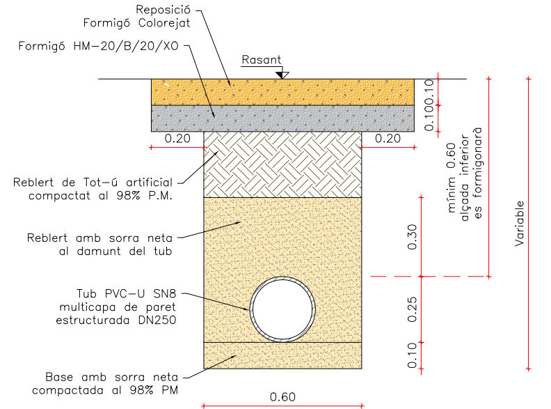
DETALL RASA CLAVEGUERAM TIPUS 4 Esc 1/20
