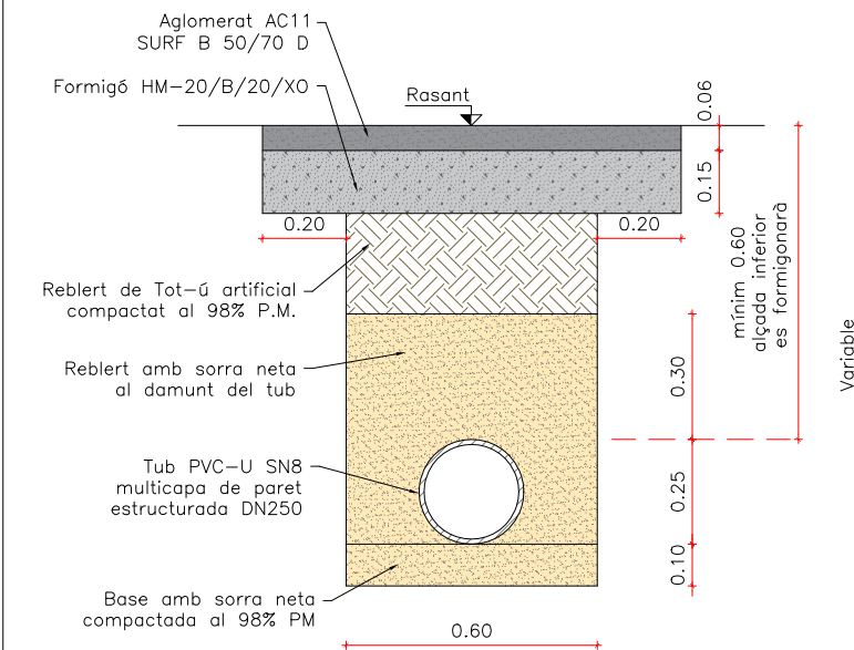
DETALL RASA CLAVEGUERAM TIPUS 1 Esc 1/20
