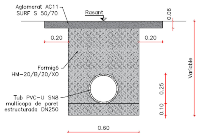
Figura 10. Detall rasa clavegueram tipus 2
