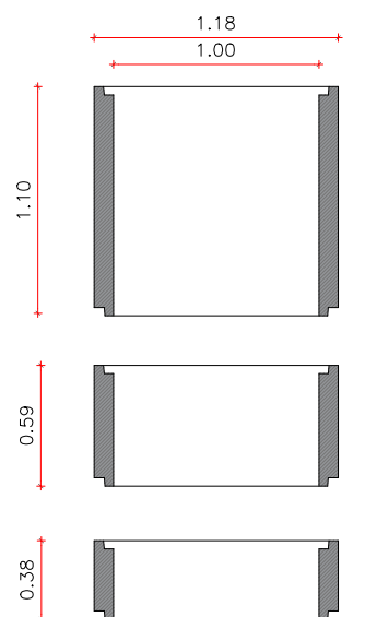
DETALL ANELLS PREFABRICATS Esc 1/40
