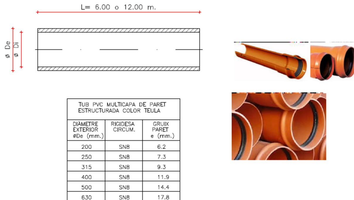
Figura 8. Detall
