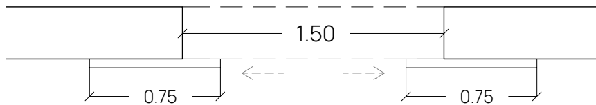
Fi 01_ Porta corredera de fusta
