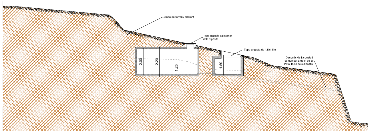
SECCIÓ A-A'
