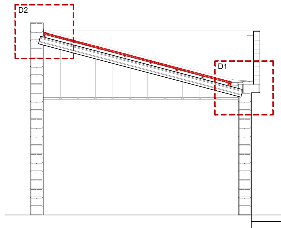
Secció proposta E:1/50
