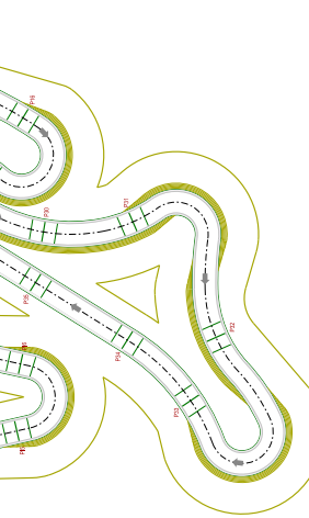
PLANTA DE PISTES DE PUMPTACK D'INICIACIÓ I PUMPTACK SUPERFÍCIE TOTAL PAVIMENTADA 1.582,63 M2 SUPERFÍCIE ZONA VORALS DE SEMBRAT NATURAL 959,14 M2 ESCALA 1/200
