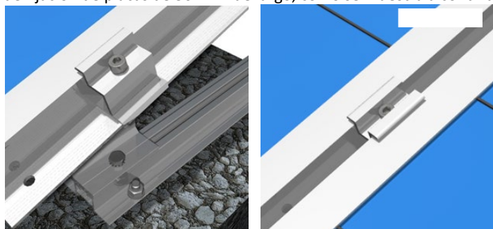
Figura 2. Detalle Brida Extremo y brida intermedia para la fijación de las placas fotovoltaicas
