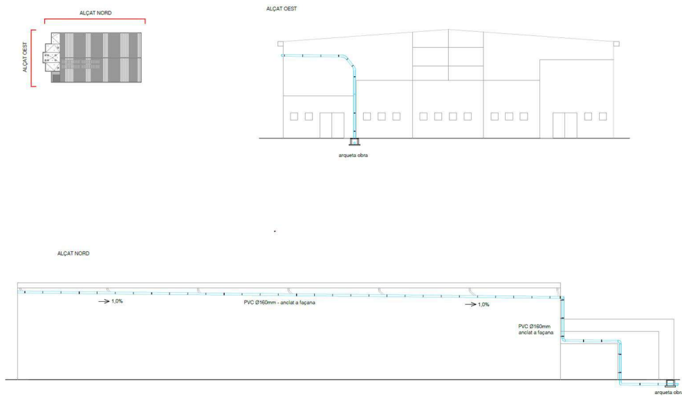
Alçats edificació. Nova actuació de recollida d'aigües pluvials
