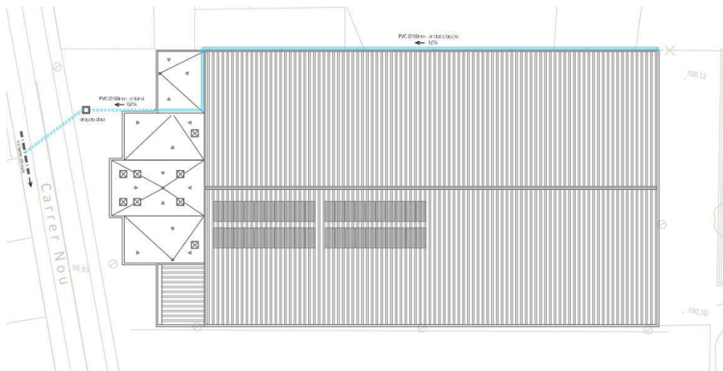
Zona exterior edificació. Nova actuació de recollida d'aigües pluvials
