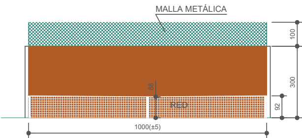
ALZADO FONDO (Dimensiones interiores)
