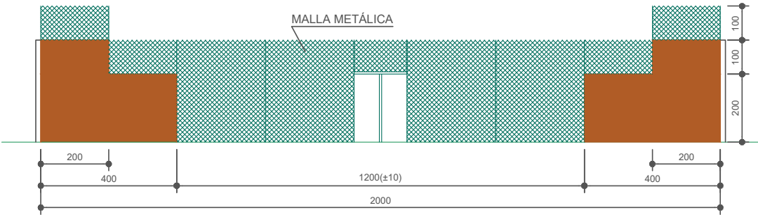
ALZADO LATERAL-variante 1 (Dimensiones interiores)
