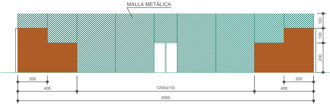
ALZADO LATERAL-variante 2 (Dimensiones interiores)
