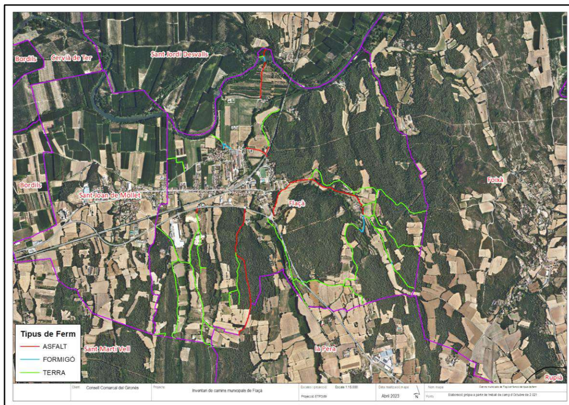
Fig. 5. Mapa de la distribució segons el tipus de ferm dels camins municipals de Flaça.
