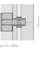
SECCIÓ B-B
