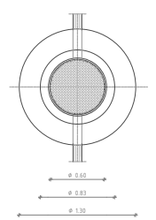
ARQUETA PER VÀLVULES DESGUASSOS I VENTOSSES PLANIF A E 1:1,40
