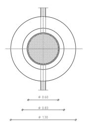
ARQUETA PER HIRPANTS D'INCENDIS seg. UNE - 23 - 103 - 81 PLANIF A E 1:1,40
