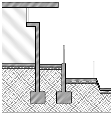
SECCIÓ B E: 1/100
