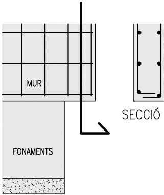
DETALL A (E: 1/25)
