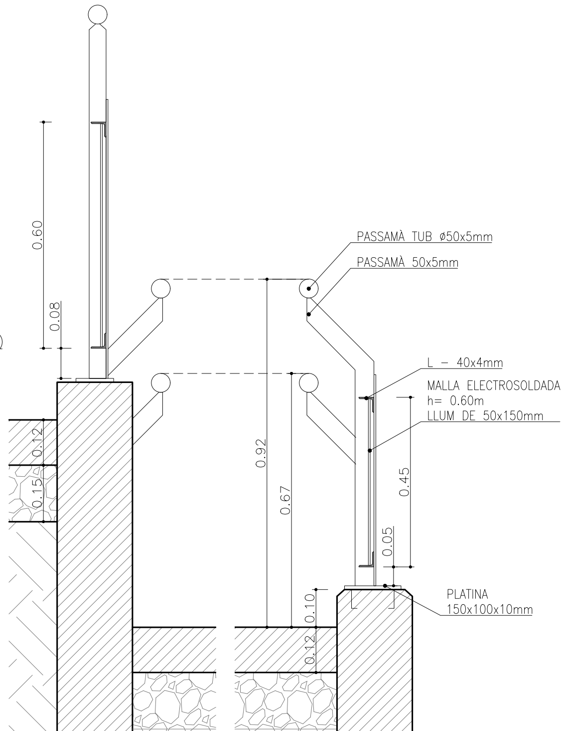
DETALL B E: 1/10
