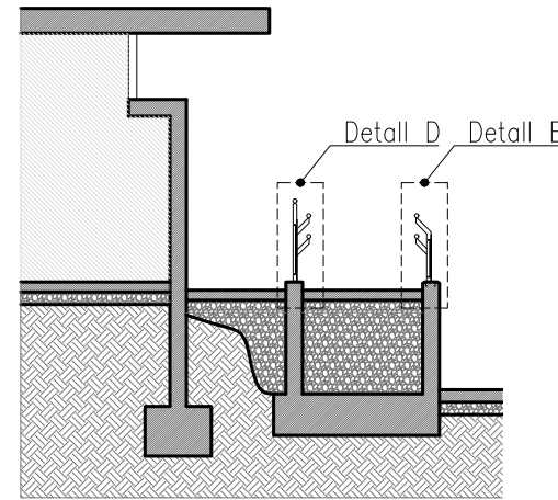
SECCIÓ C E: 1/100
