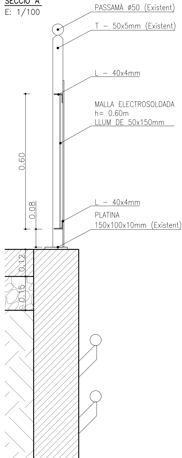
DETALL A E: 1/10
