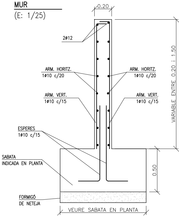
DETALL A (E: 1/25)
