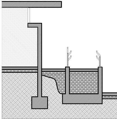
SECCIÓ C E: 1/100
