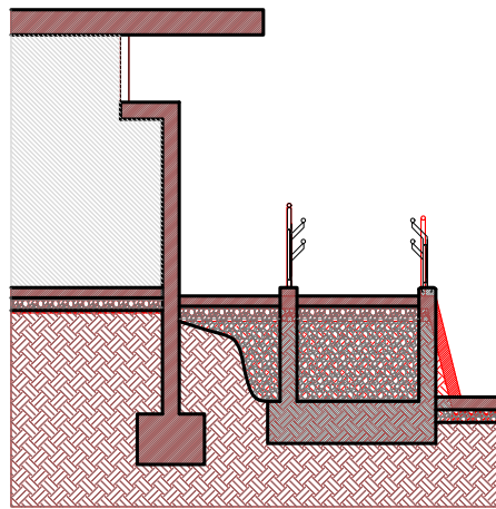
SECCIÓ C
