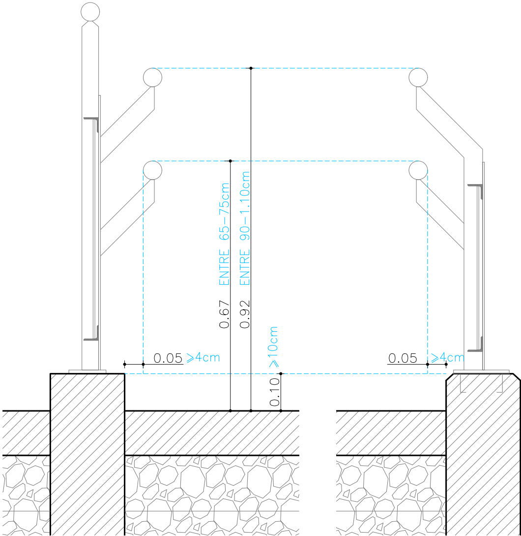
DETALL ACCESSIBILITAT E: 1/10
