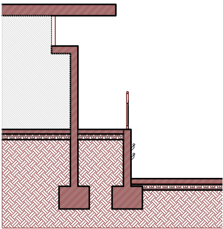
SECCIÓ A
