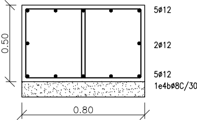
SABATA S-03 (E: 1/25)
