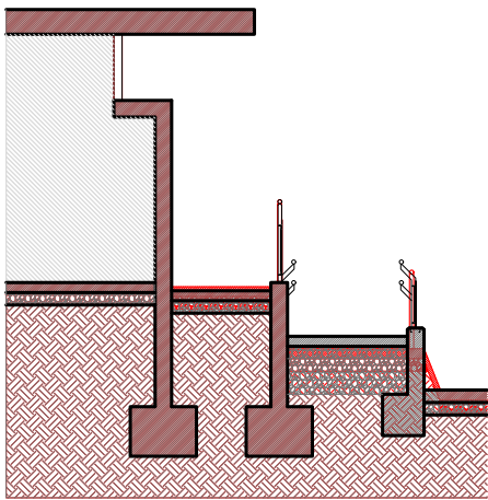
SECCIÓ B
