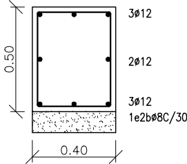
SABATA S-01 (E: 1/25)
