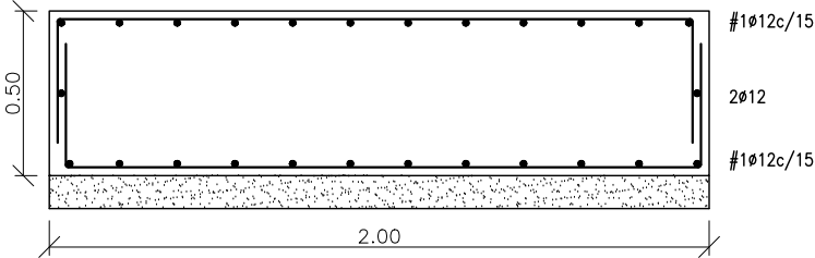
SABATA S-04 (E: 1/25)
