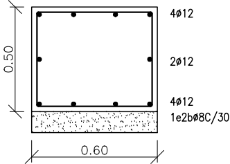
SABATA S-02 (E: 1/25)
