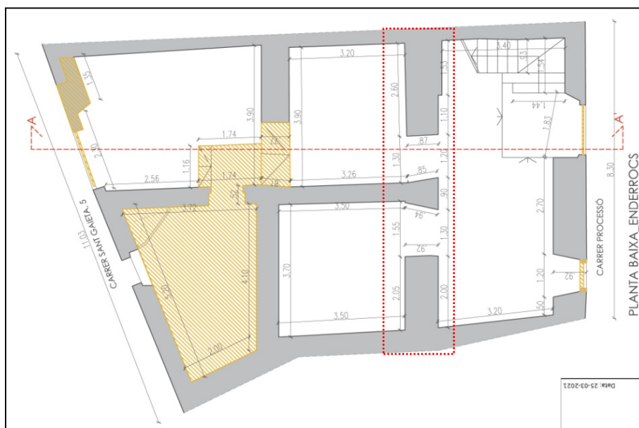
Planta baixa del projecte de rehabilitació de l'edifici situat al carrer de Sant Gaietà, 5 i situació del mur que coincideix amb el traçat de la muralla.
