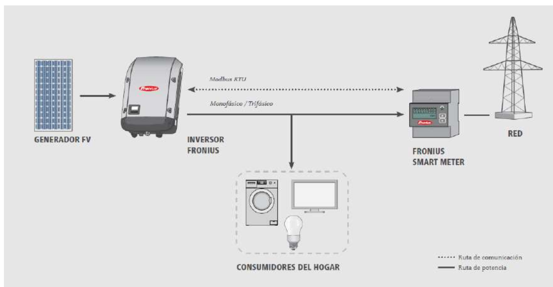
Fig. 11. Connexió del sistema Smart Meter de Fronius
