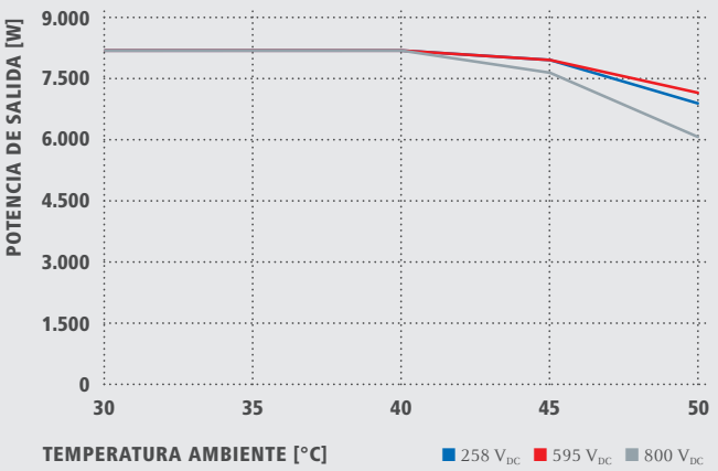
REDUCCIÓN DE TEMPERATURA FRONIUS SYMO 8.2-3-M
