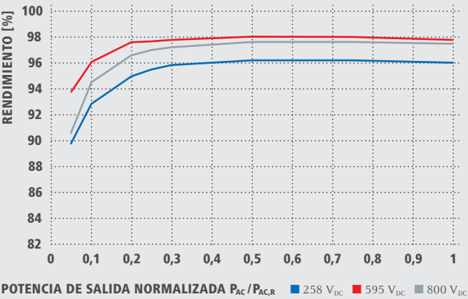
CURVA DE RENDIMIENTO FRONIUS SYMO 8.2-3-M
