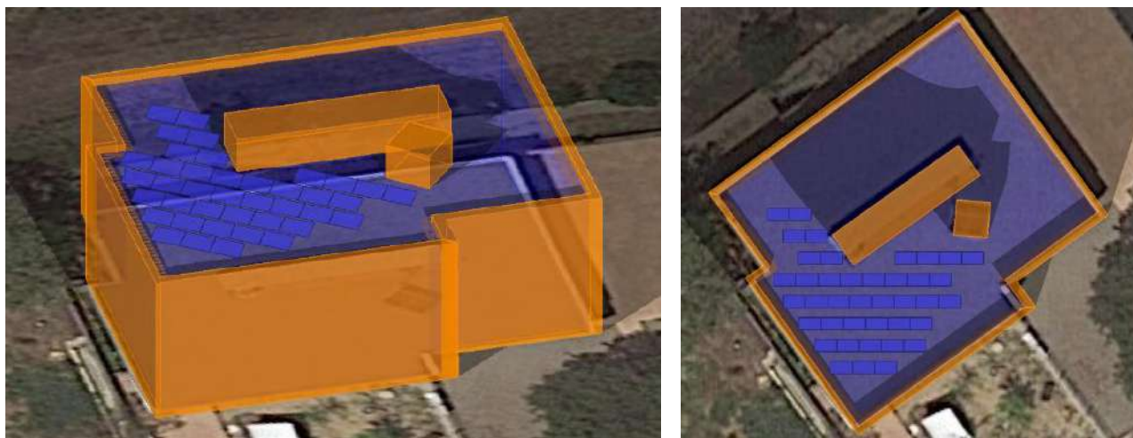
Fig. 6. Simulació de l'afectació d'ombres projectades sobre la instal·lació fotovoltaica
